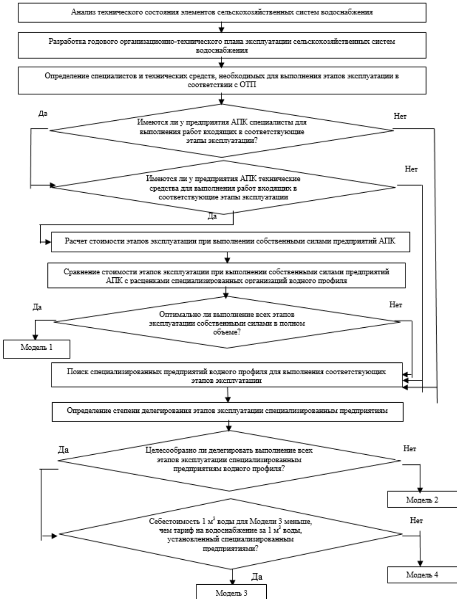
Рис. 2. Алгоритм принятия решений по выбору оптимальной организационной модели эксплуатации сельскохозяйственных систем водоснабжения (Далее – Алгоритм)
